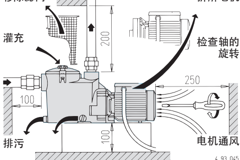
图1 最小检修尺寸
