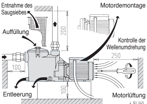
Abb. 1 Mindestraumbedarf für Wartung (mm)
