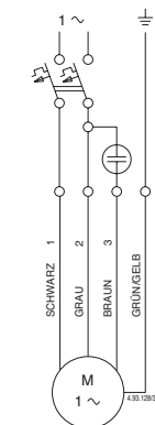
Schaltbild Einphasen-Wechselstrommotoren
