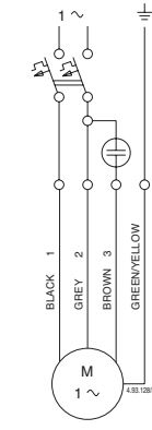
Ηλεκτρικό σχεδιάγραμμα
