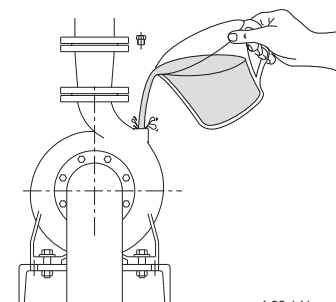
Рис. 3 Заполнение жидкостью
