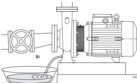
Рис. 4 Слив воды
